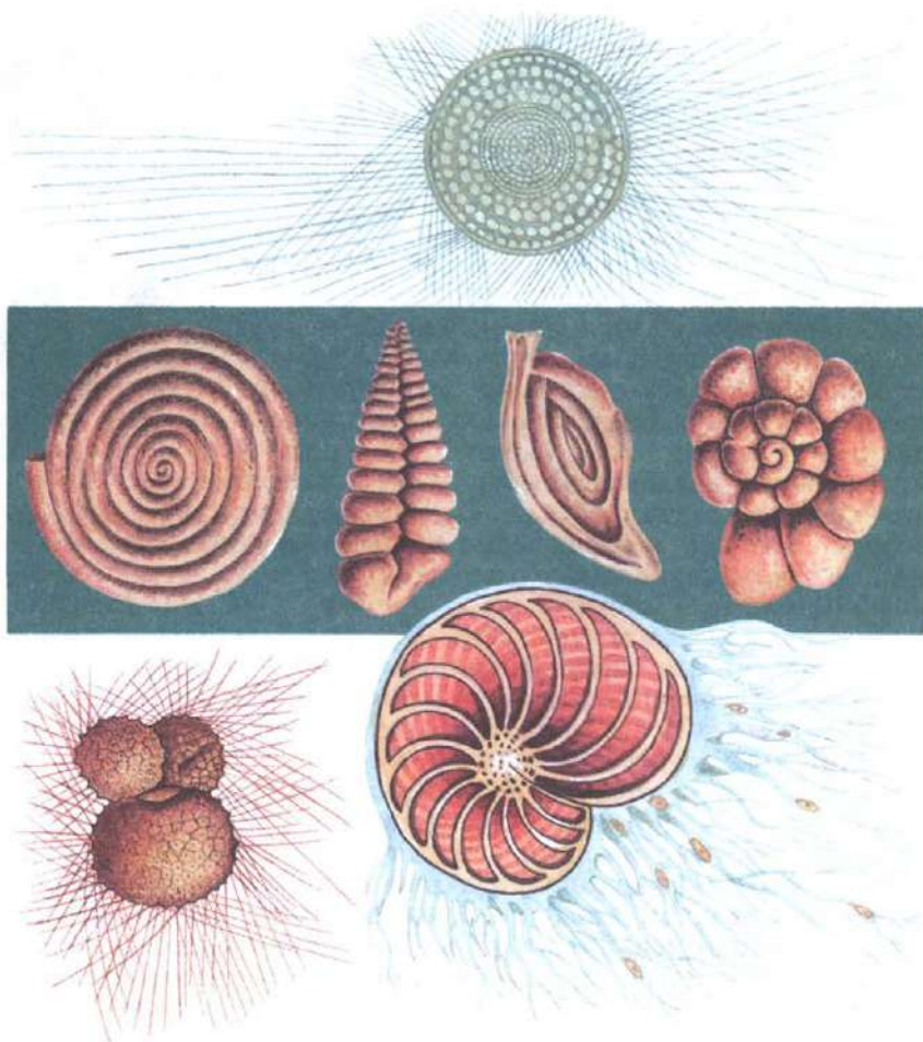
Рис. 79. Фораминиферы.
